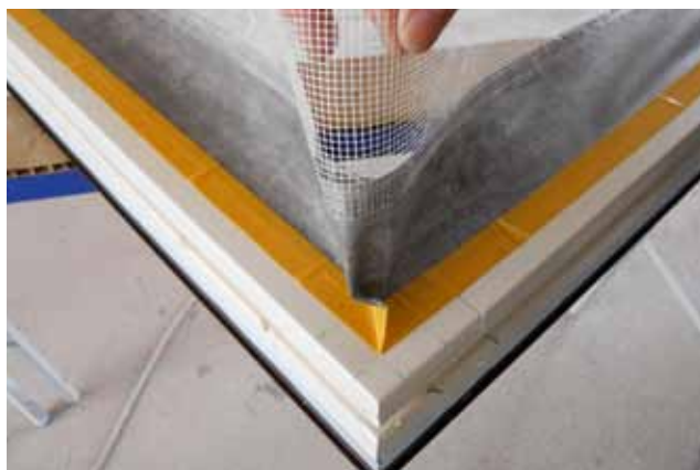
Posa di bandella per la tenuta all'aria sul telaio del serramento.
